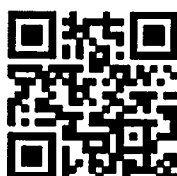
QR Code 2
